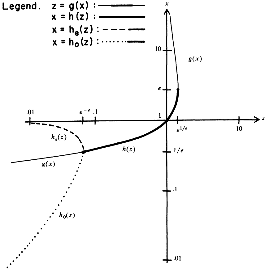
FIG. 4. z^{z^z} = z
